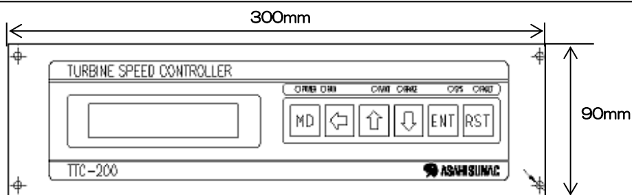
図9 TTC200 外観図
