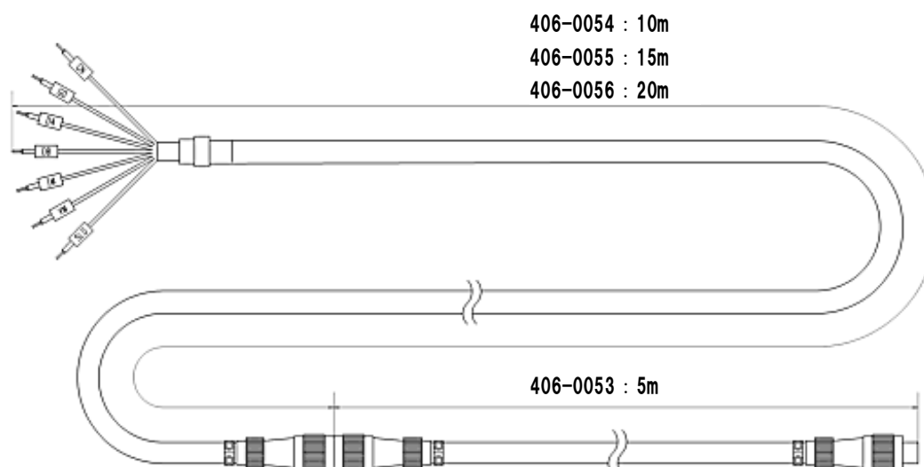
図5 送電ケーブル接続図
