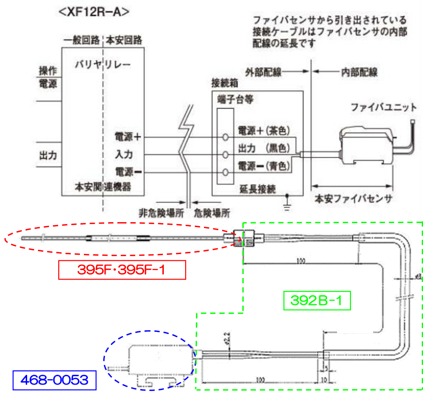
図7-2 防爆仕様光ファイバーケーブル接続図
