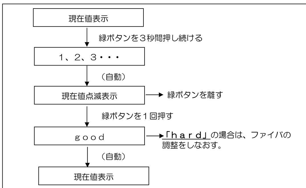
【参考】光ファイバアンプオートチューニングフロー
