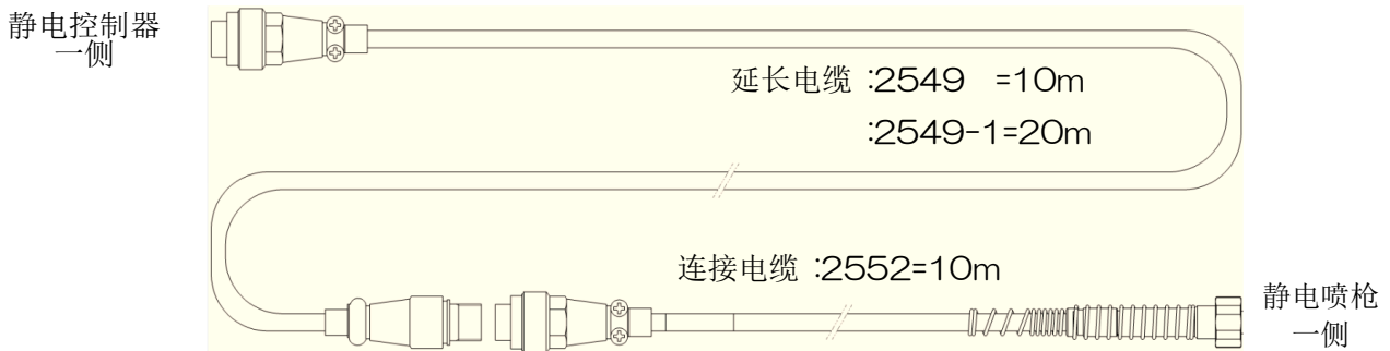
输电电缆连接图
