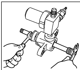
⑩ピストンロッド⑤にスパナを掛け、チェックバルブ⑥のネジ部をはずし、Vパッキンと一緒にチェックバルブをはずす。
