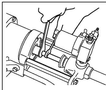
⑧ナット(⑪, ⑫)をゆるめ、ロッドとピストンロッド⑤とのネジ部をはずし、エアモータ部とマテリアルシリンダ部を切り離す。
