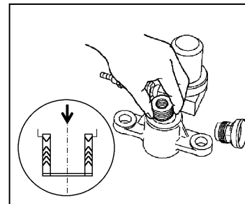
⑫新しいパッキンを1枚ずつ入れる。(この時パッキン当金④とV型パッキンの向きに注意して反対方向に入れないようにしてください。)
