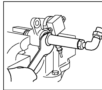
⑨ポンプハウジング①からシリンダ⑫をはずす。
