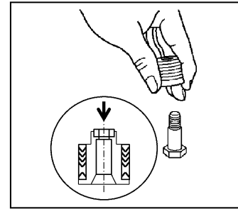
⑮新しいパッキンを1枚ずつ入れる。(この時パッキン当金④とV型パッキンの向きに注意して反対方向に入れないようにしてください。)
