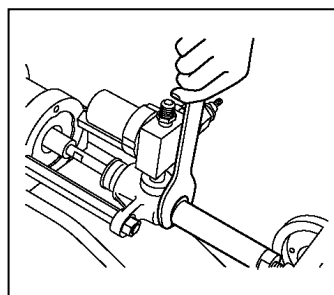
⑬ポンプハウジング①からシリンダ⑫をはずす。
