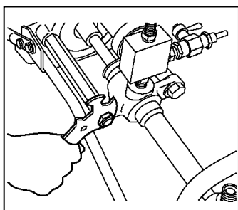
⑦マテリアルホースをはずした後、ポンプハウジング①を接続するステイの締付ナットをはずす。
