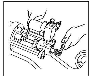
⑭ピストンロッド⑤にスパナを掛け、チェックバルブ⑥のネジ部をはずし、チェックバルブと一緒にVパッキンをはずす。
